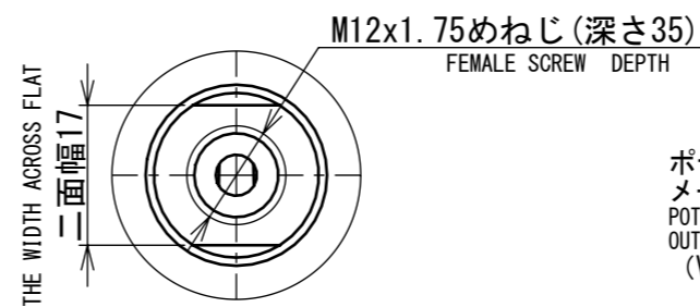
詳細図 B DETAIL VIEW B
