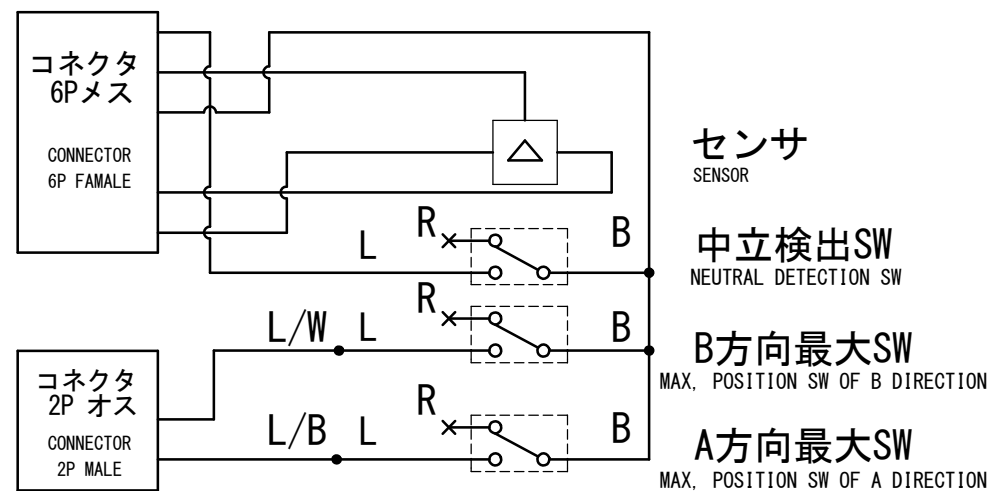
配線図 CIRCUIT DIAGRAM
