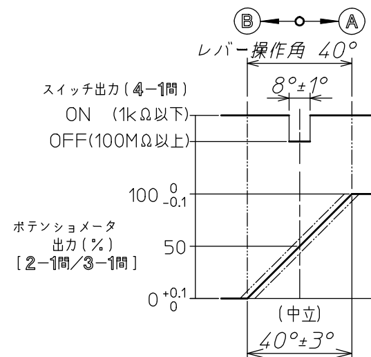
ポテンシオメータ出力特性
