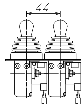
レバー取付けピッチ
