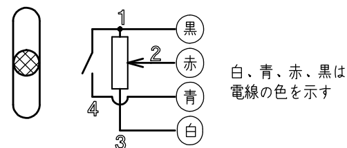
配線図
