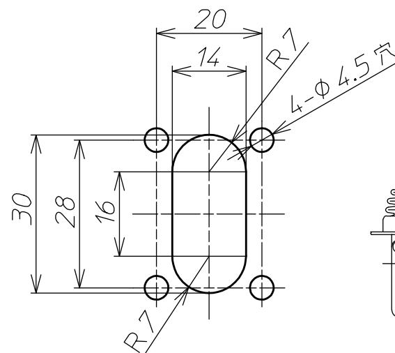
パネル面取付穴，寸法指示図
