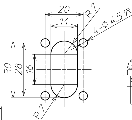
パネル面取付穴，寸法指示図
