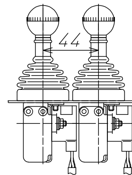
レバー取付けピッチ
