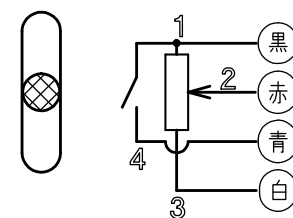
配線図
