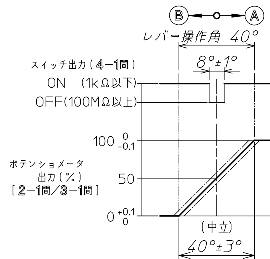
ポテンショメータ出力特性
